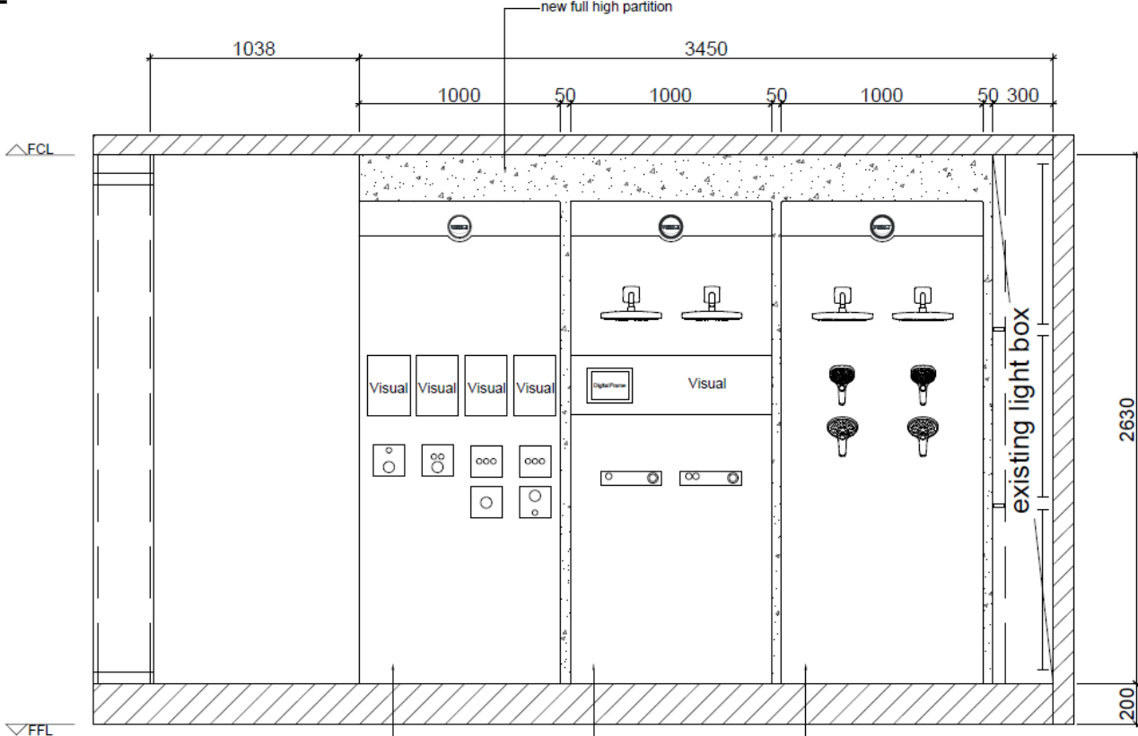
ELEVATION C SCALE: 1:20
