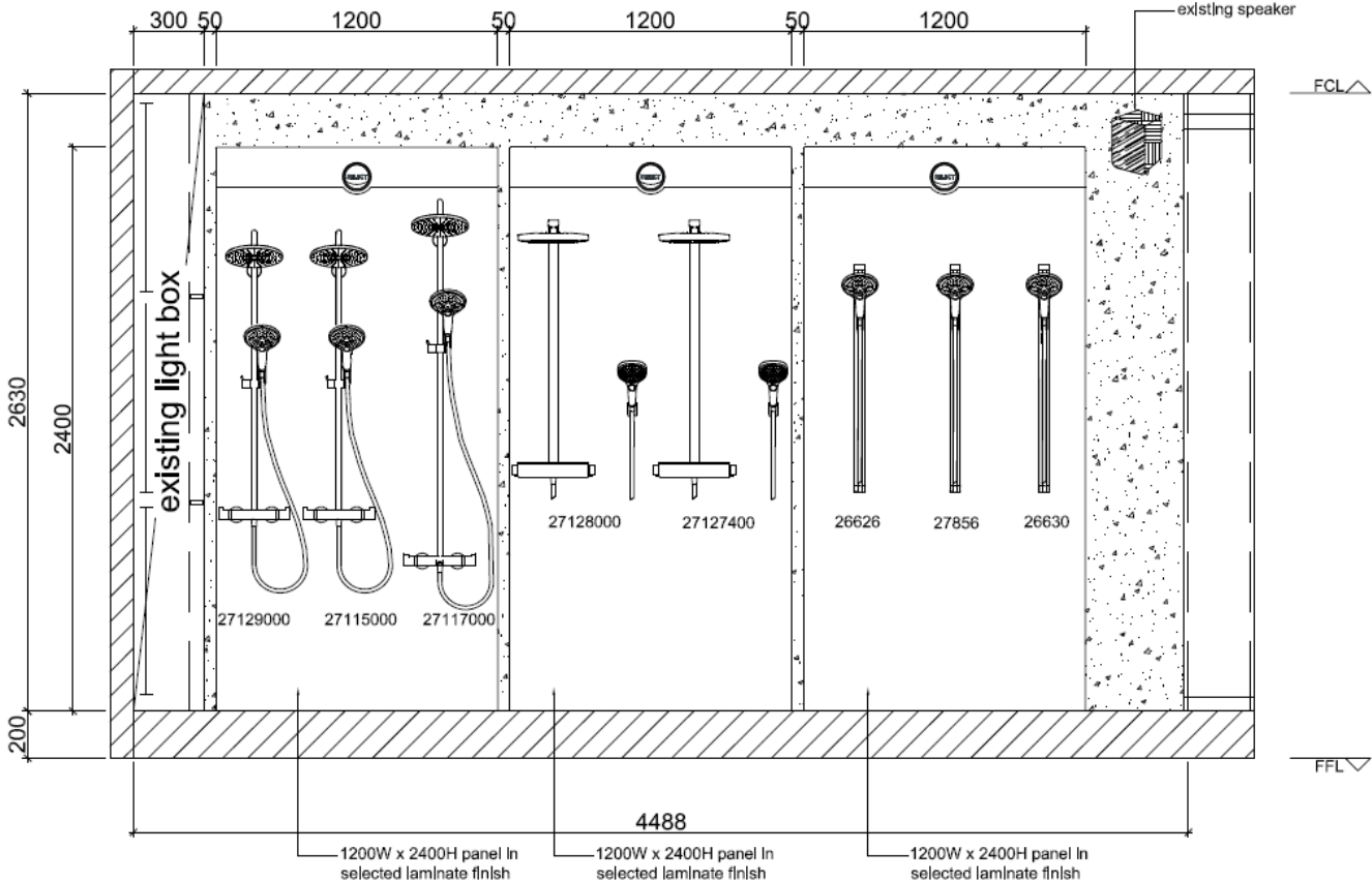
ELEVATION B SCALE: 1:20
